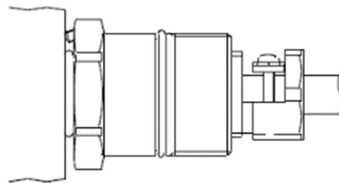
図8-2: 座金、シーリング部拡大図
