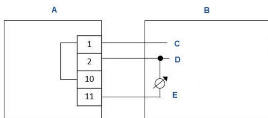
図3-9:ソース3線式
